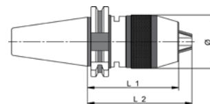
DIN-69871-A
