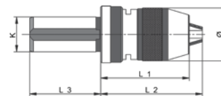
DIN-69893-A [HSK]
